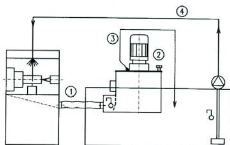
Principskiss över reningsflödet i T14 kopplad med maskin och tank.
